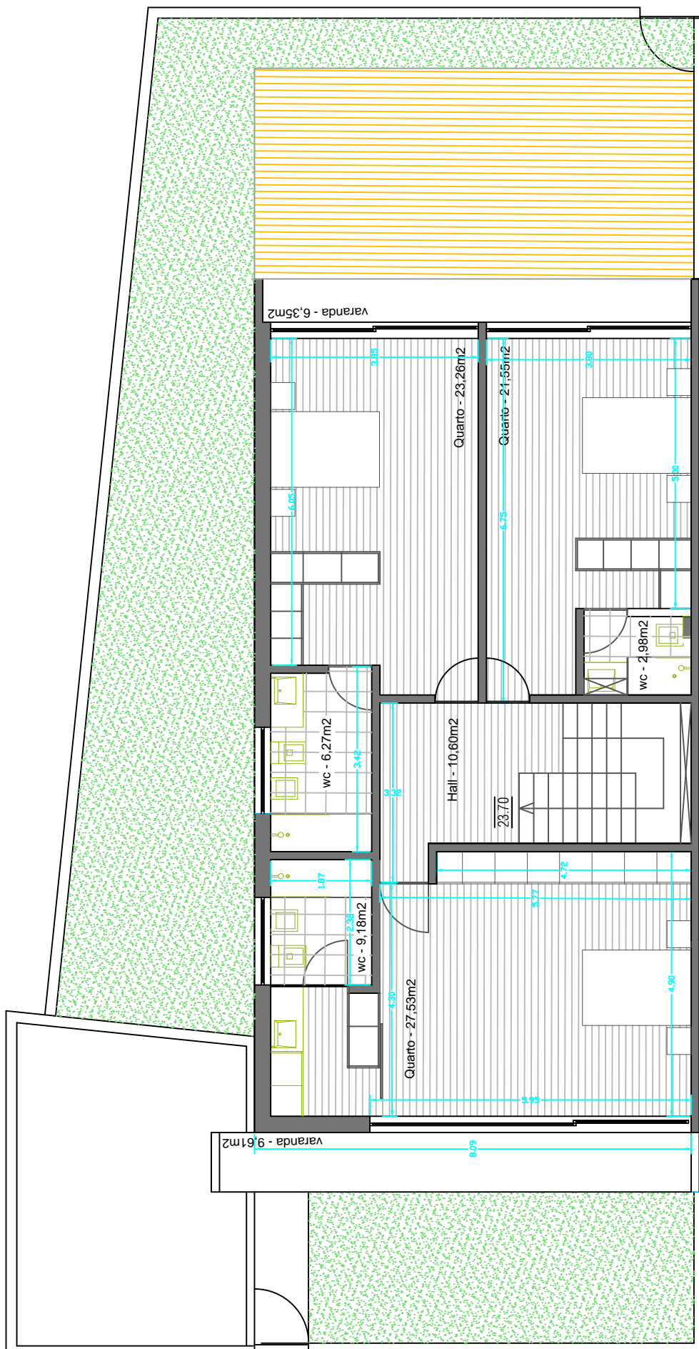
Planta Piso 1
